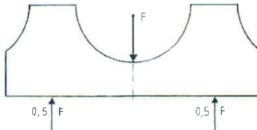
Bild 1: Belastungsanordnung Biegeversuch
