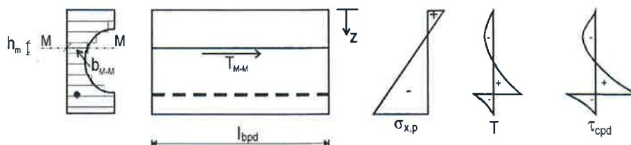
Bild 1: Ermittlung der Schubspannung aus Spannkrafteinleitung
